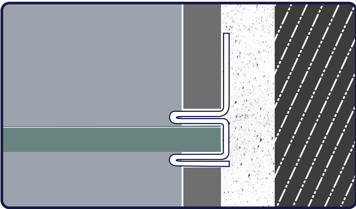
Vertical Installation on Wall Instalación Vertical en la Pared
