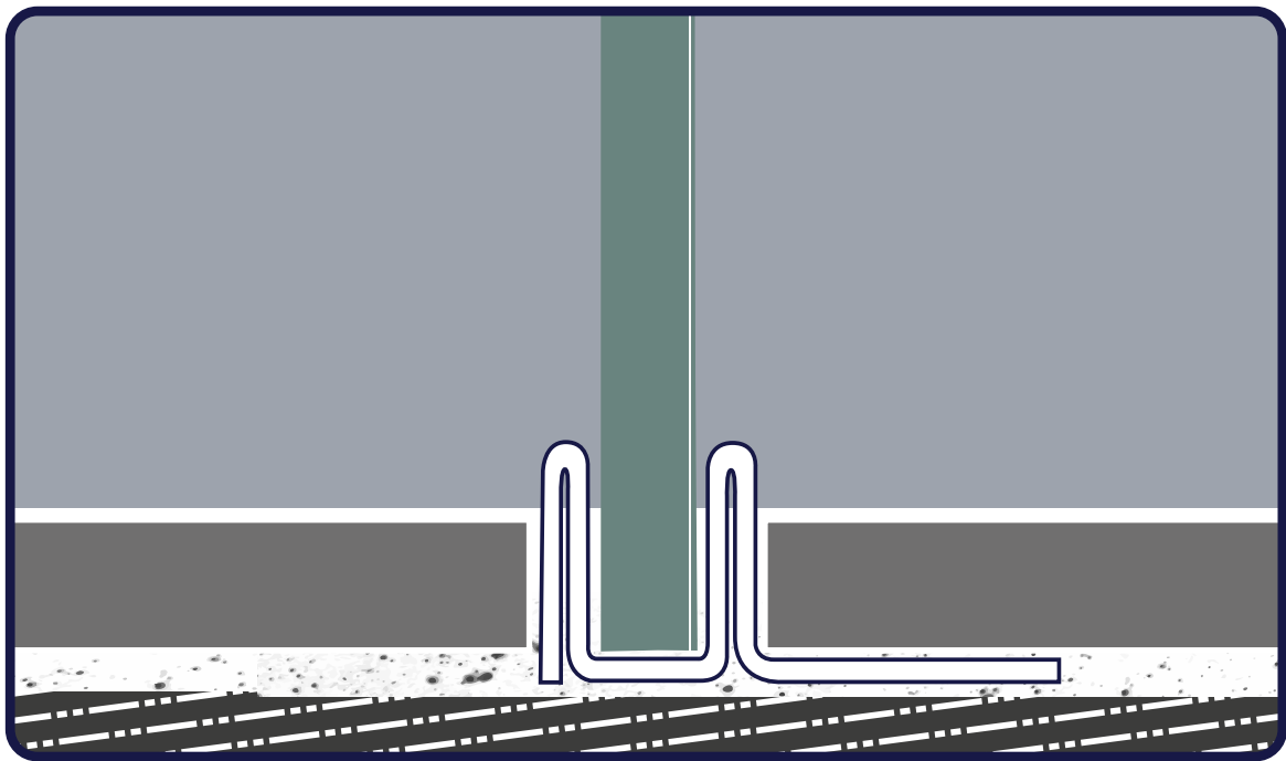
Horizontal Installation on Flooring Instalación Horizontal en Pavimento
